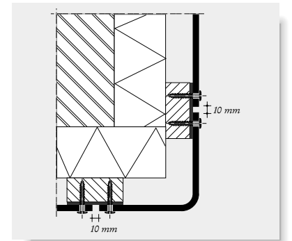
Trespa-Eckelement
