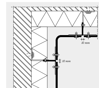
Trespa-Eckelement
