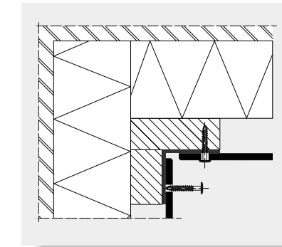
Innenecke
