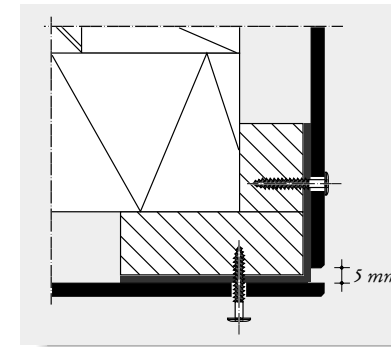
Aussenecke
